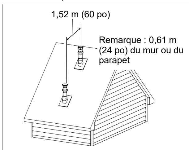
Figure 12 : Entre des extrémités à différents niveaux
