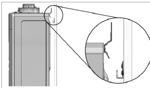
Figure 6 : Fixer le crochet supérieur
