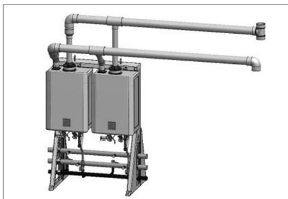
Figure 37 : Exemple de configuration sur pied, en série
