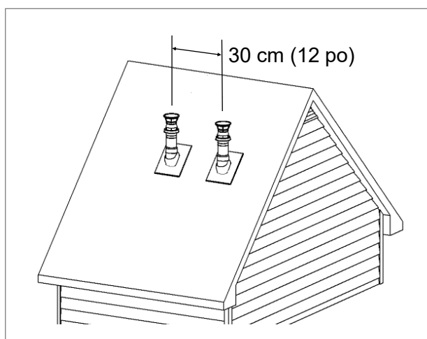
Figure 13 : Entre des extrémités au même niveau
