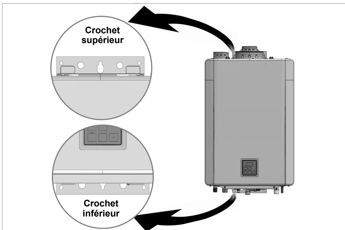
Figure 7 : Crochets supérieur et inférieur
