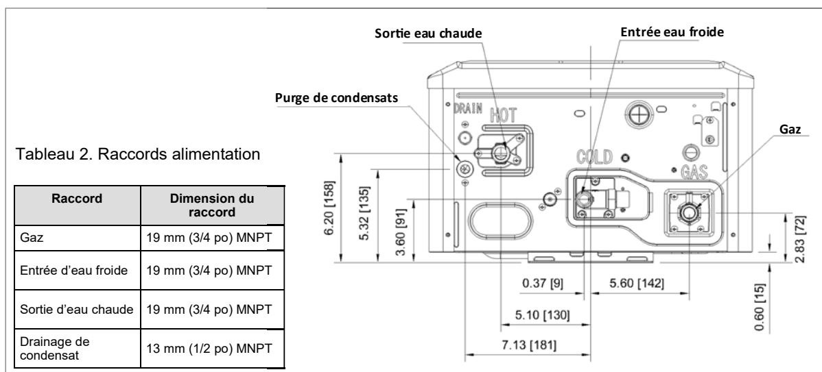
Figure 3 : Raccords d'alimentation
