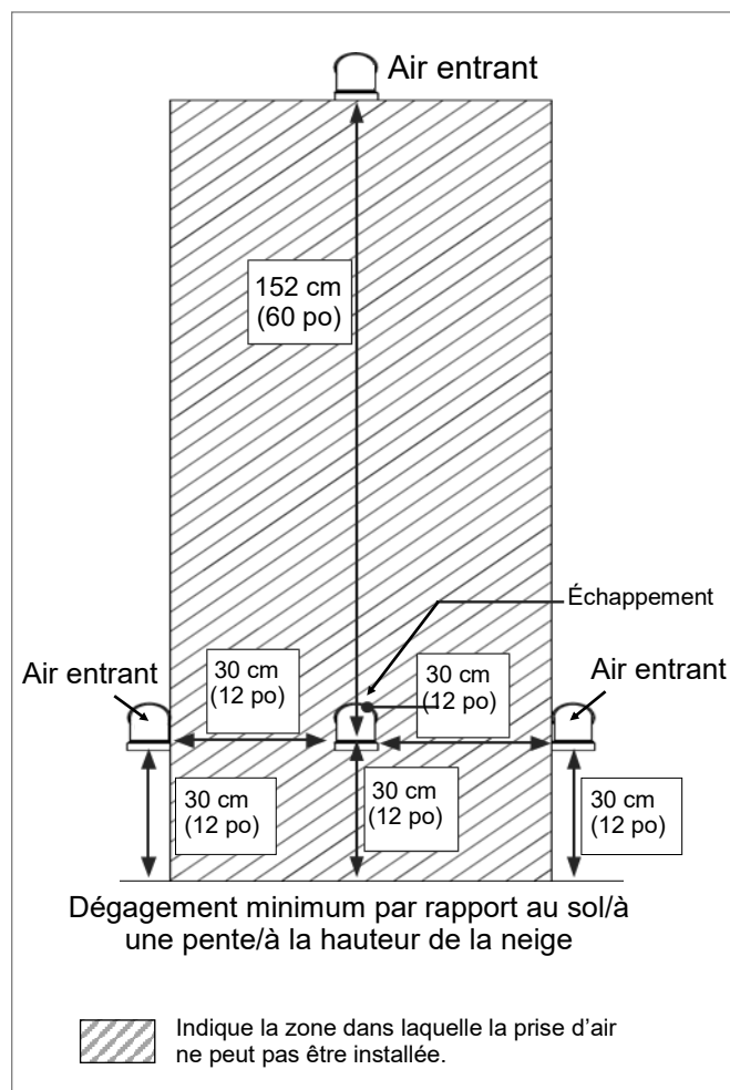
Figure 21 : Conduit d'évacuation horizontal et tuyauterie d'air entrant
