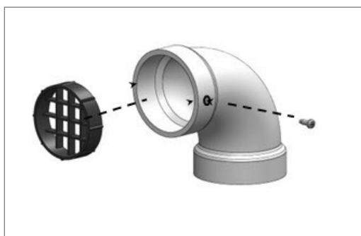
Figure 8 : Grille d'évacuation
