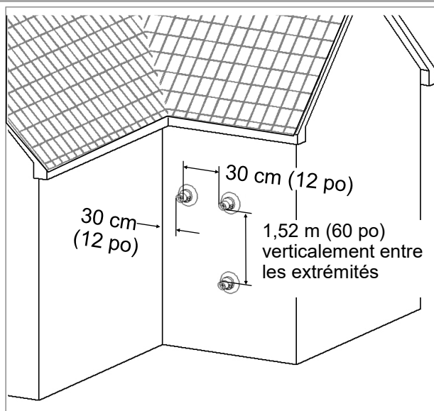
Figure 11 : Dégagements de l'extrémité du conduit concentrique
