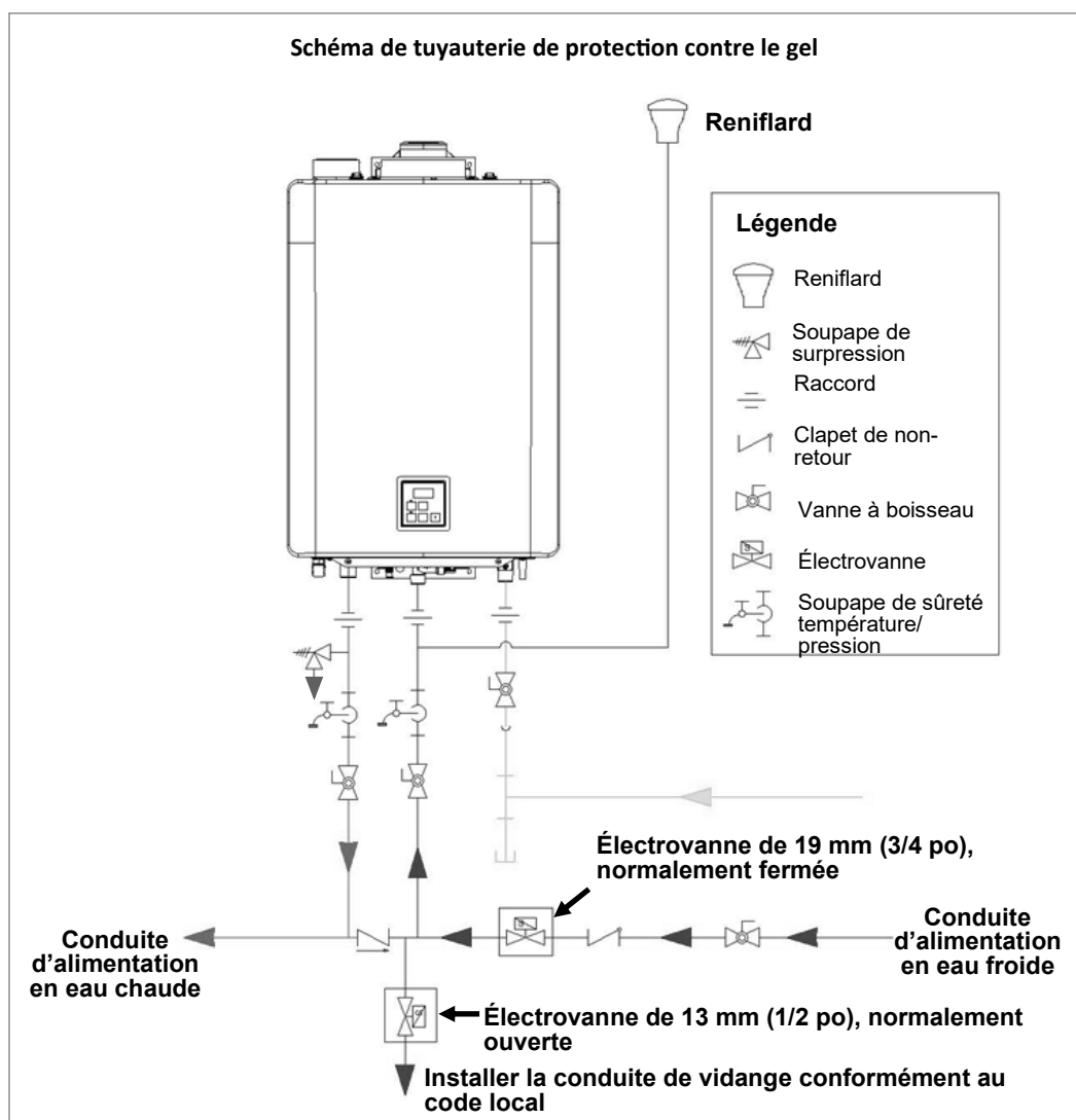
Figure 4 : Schéma de tuyauterie de protection contre le gel
