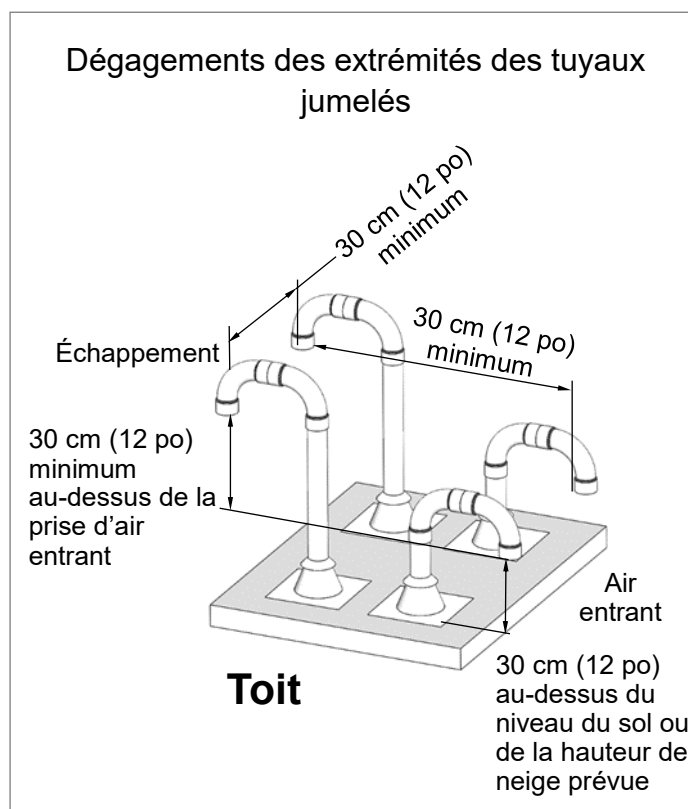
Figure 20 : Extrémités verticales des tuyaux jumelés de plusieurs chauffe-eau
